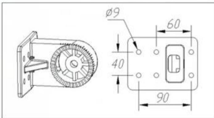
F2 Bracket
