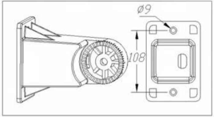
D2 Bracket
